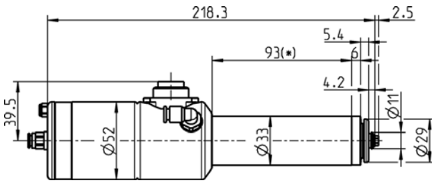
寸法図
