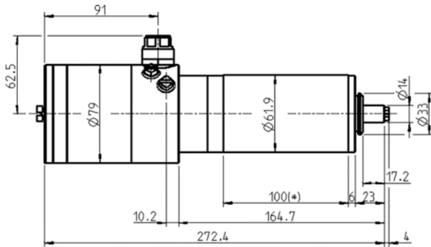
寸法図
