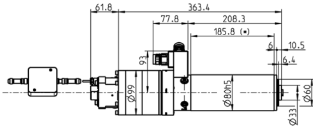
寸法図
