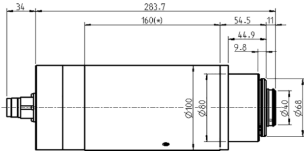
寸法図
